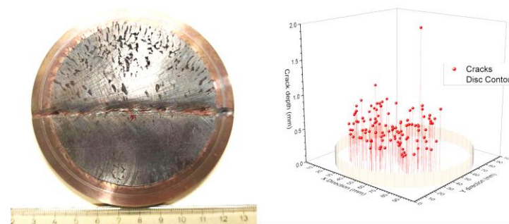
浜岡 5 号機の腐食試験
