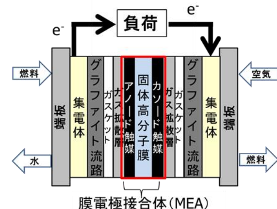
燃料電池の模式図
