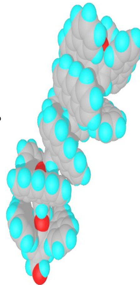
光エネルギー伝達分子
